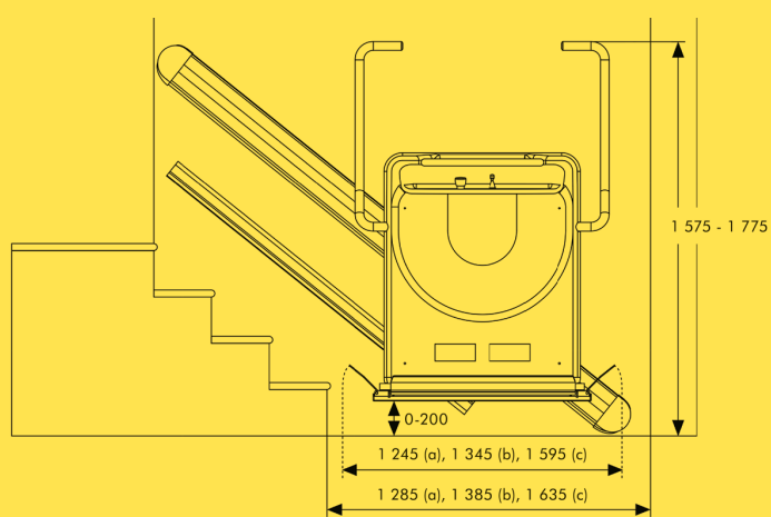
VUE DE FACE : DÉPART VERTICAL (OPTION)
