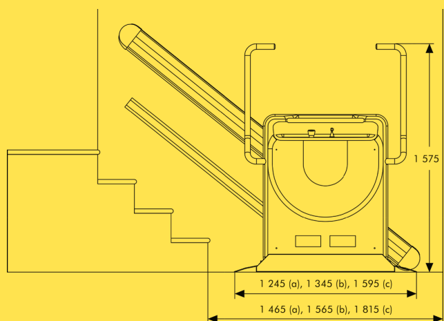
VUE DE FACE : DÉPART OBLIQUE (STANDARD)
